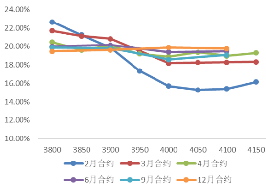
图 2.6: 沪深 300 股指期权波动率微笑
