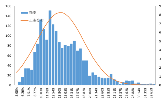
图 3: 豆粕期货历史波动率正态分布 (20HV)
