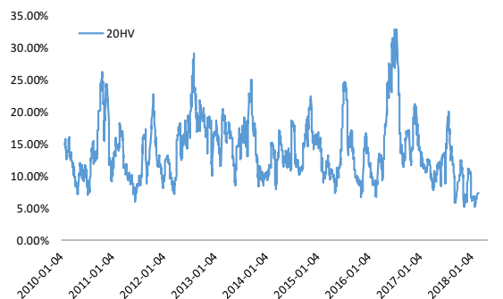
图 4: 豆粕期货历史波动率 (20HV)
