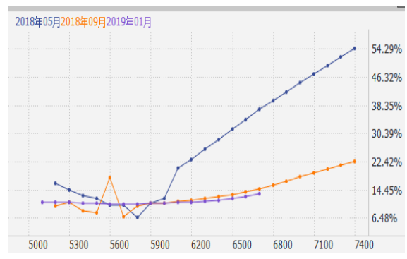
图 7: 白糖看跌期权 Volatility smiles
