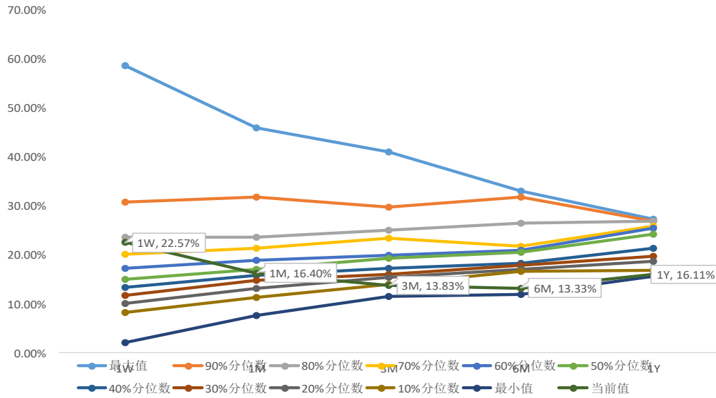
图5: 豆粕波动率锥
