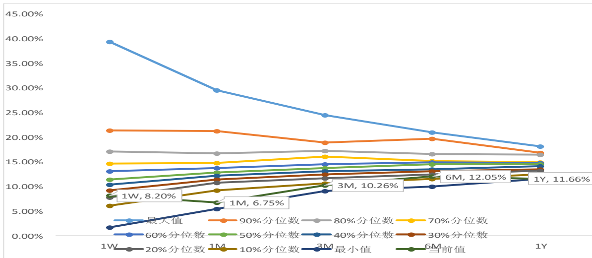
图10: 白糖波动率锥
