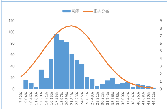
图 8: 白糖期货历史波动率正态分布 (20HV)
