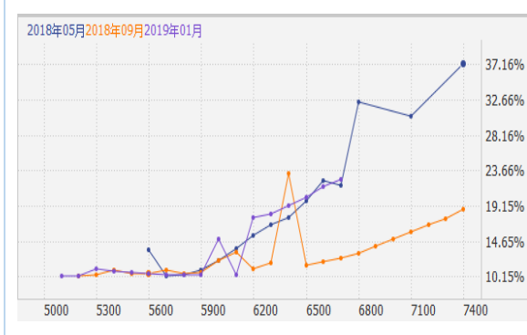
图 6: 白糖看涨期权 Volatility smiles
