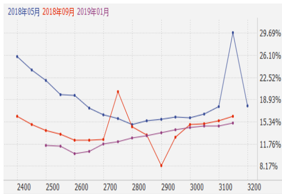
图 4: 豆粕期货历史波动率 (20HV)
